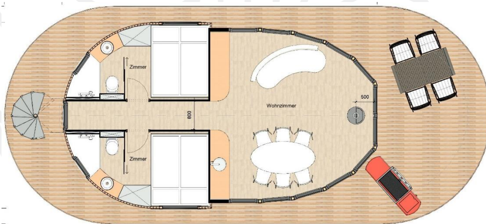
Beispielgrundriss mit ca. 5,70 m Breite und umlaufendem Gangboard (Das Basisboot ist 5,10 m breit und somit für mehr Schleusen geeignet)
